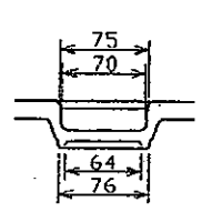
B-B断面
