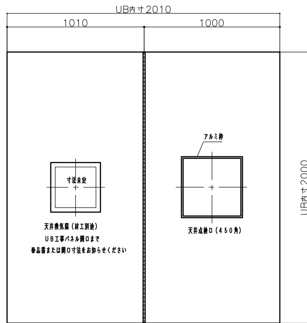
天井伏図
