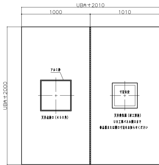
天井伏図
