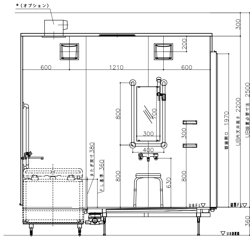
A面
