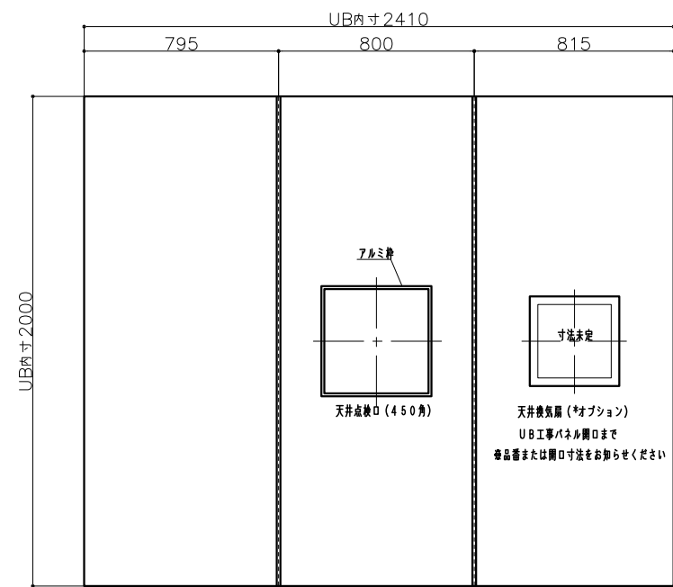
天井伏図
