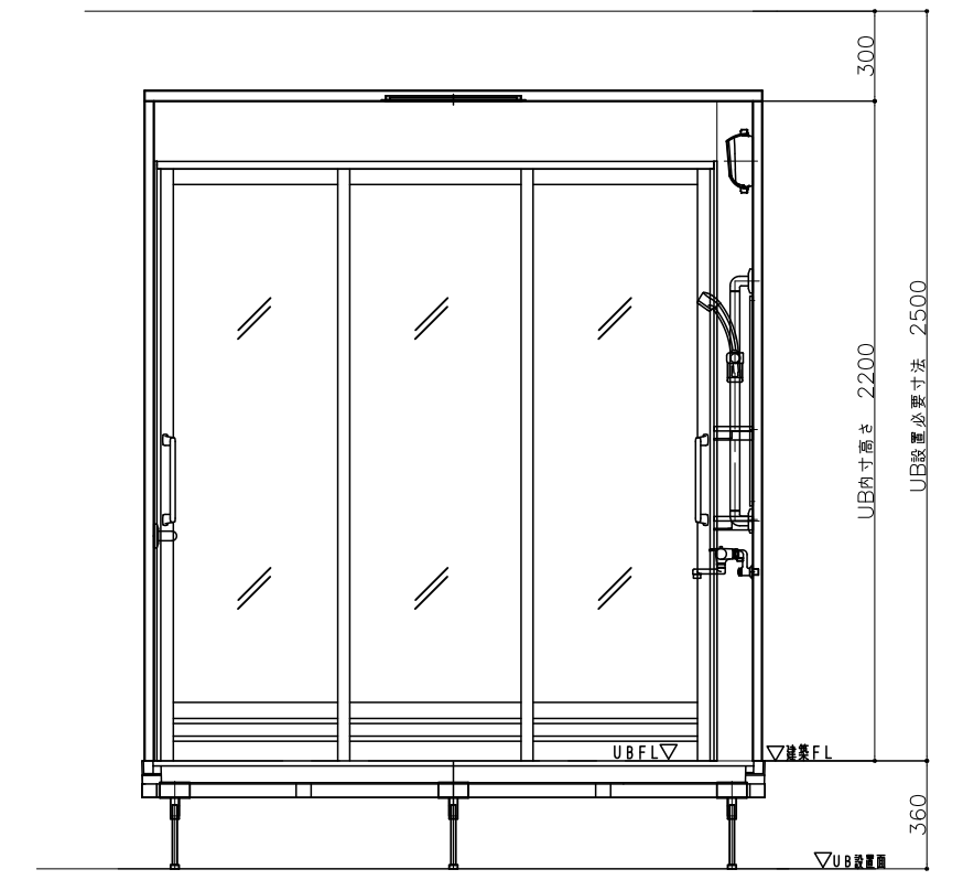
D面
