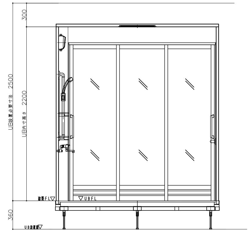
B面
