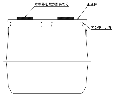
水準器のあて方
