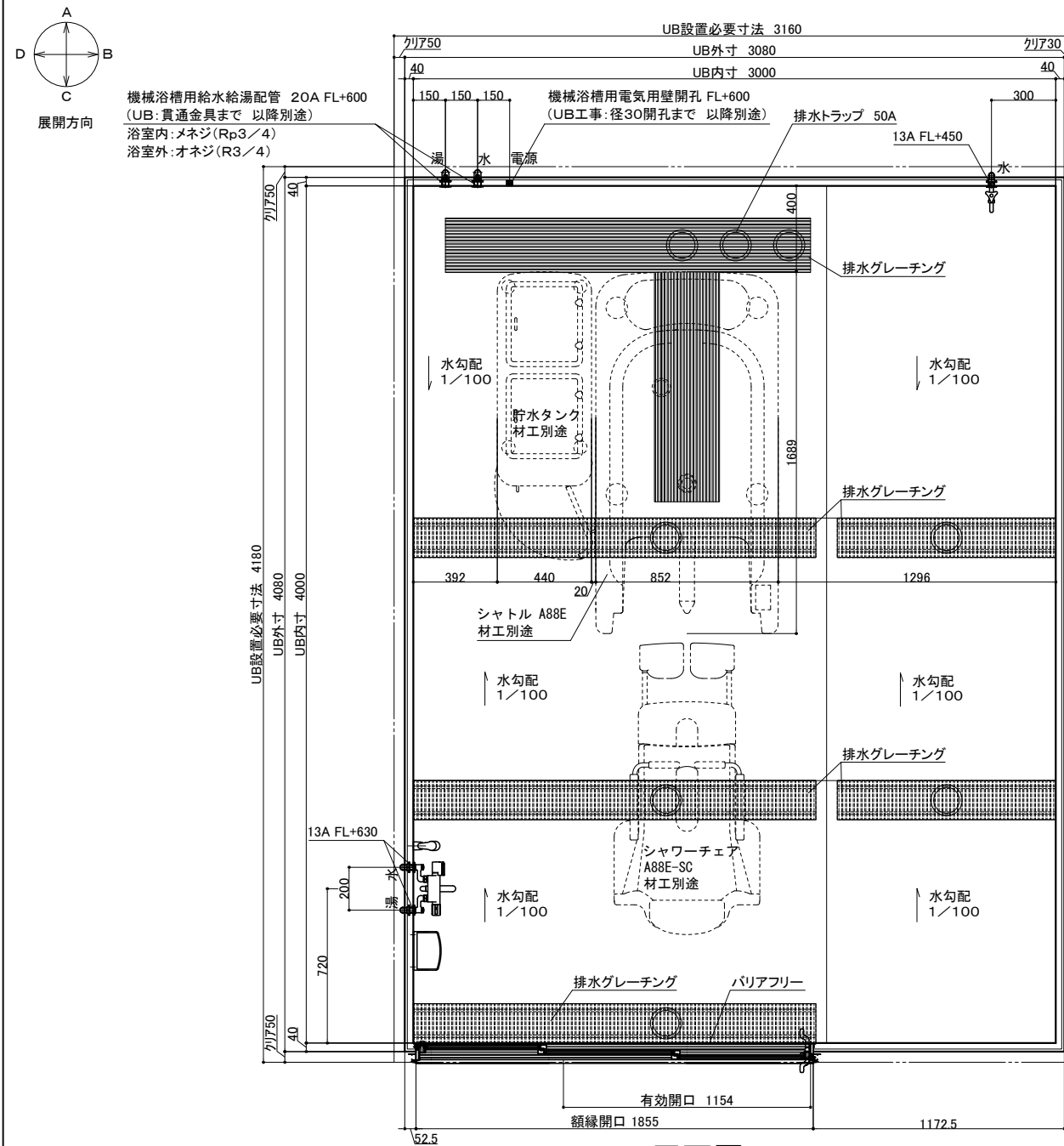
平面図
