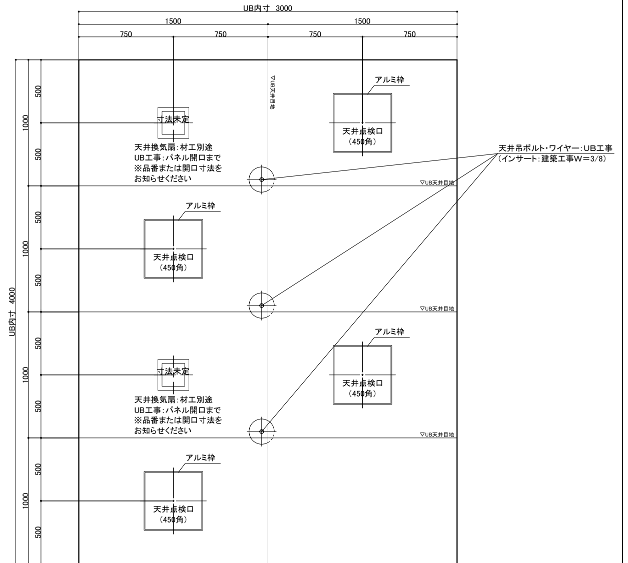
天井伏図
