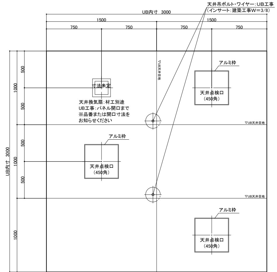
天井伏図
