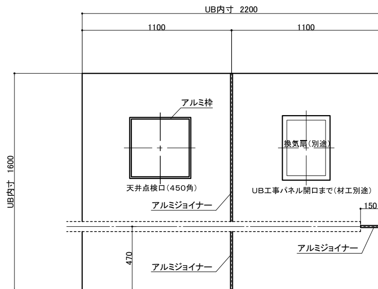
天井伏図
