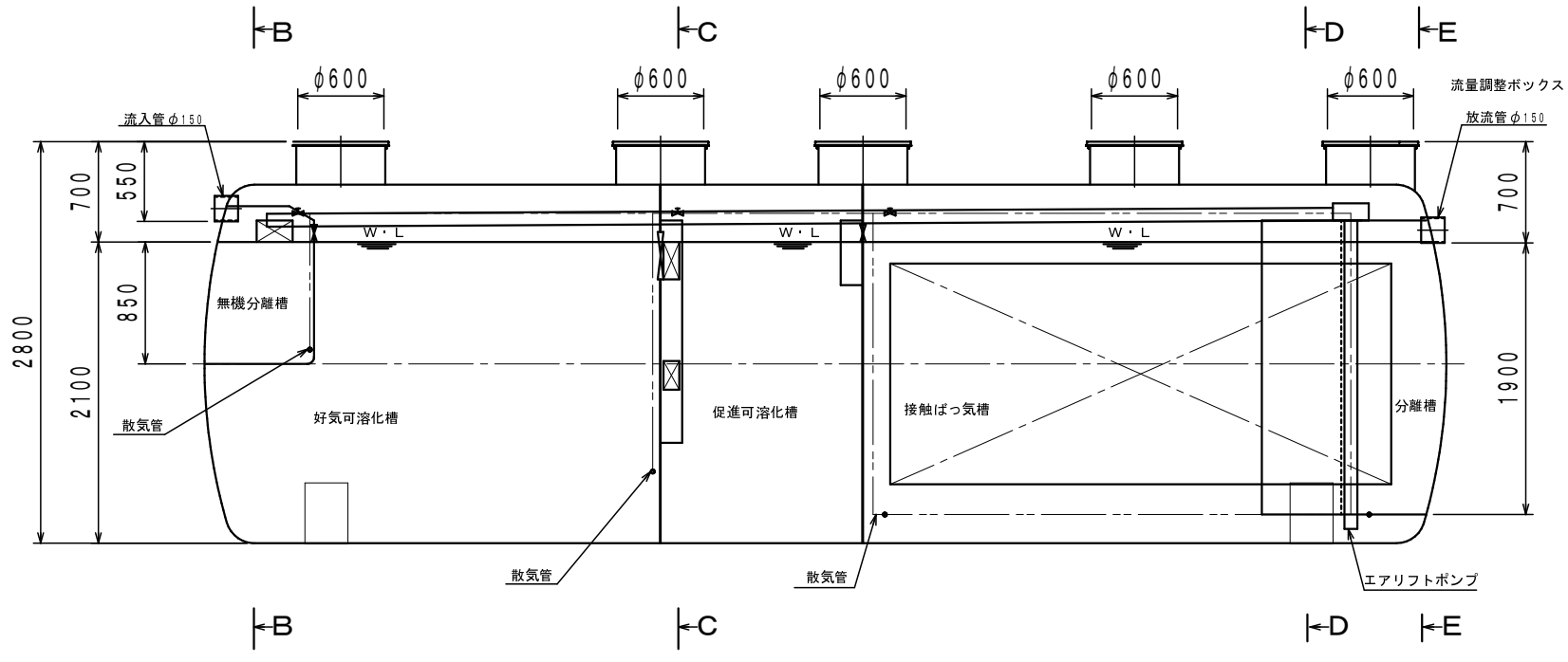
A-A断面
