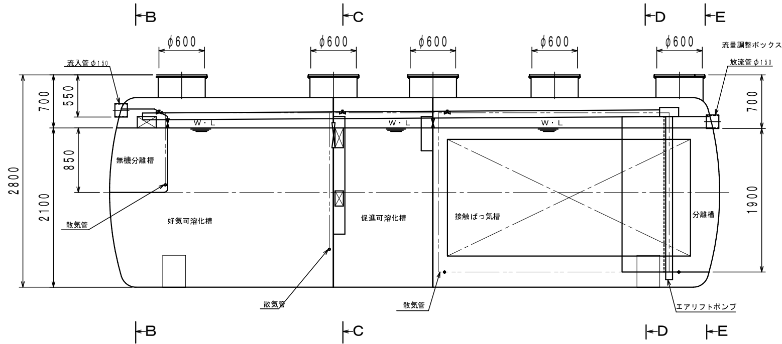
A-A断面
