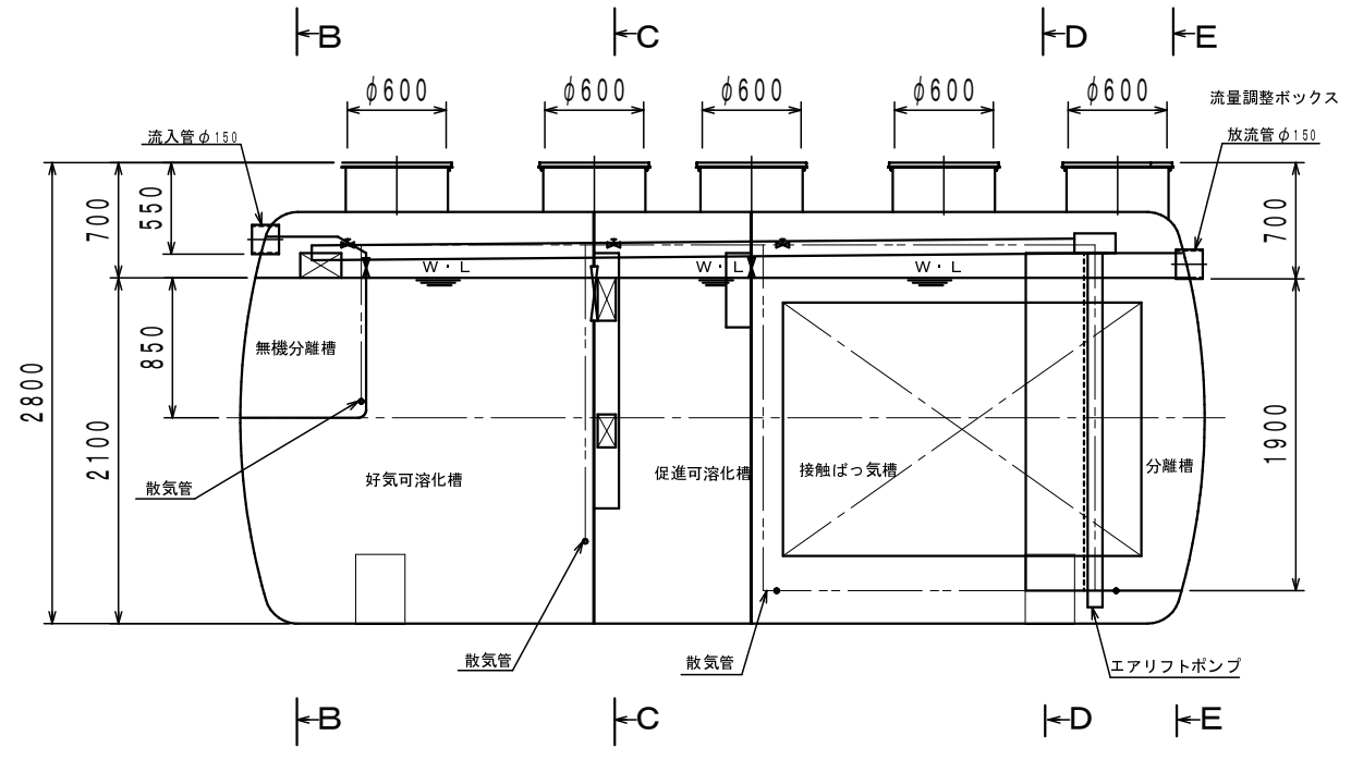
A-A断面
