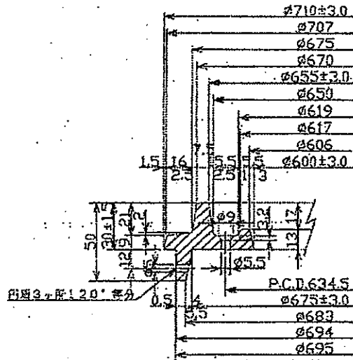
断面 B-B
