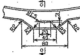
C-C詳細
