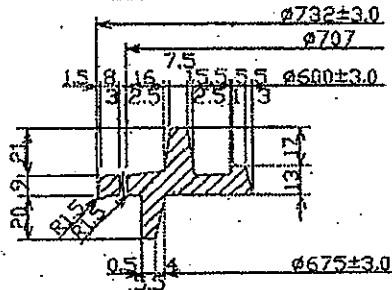
断面 C-C
